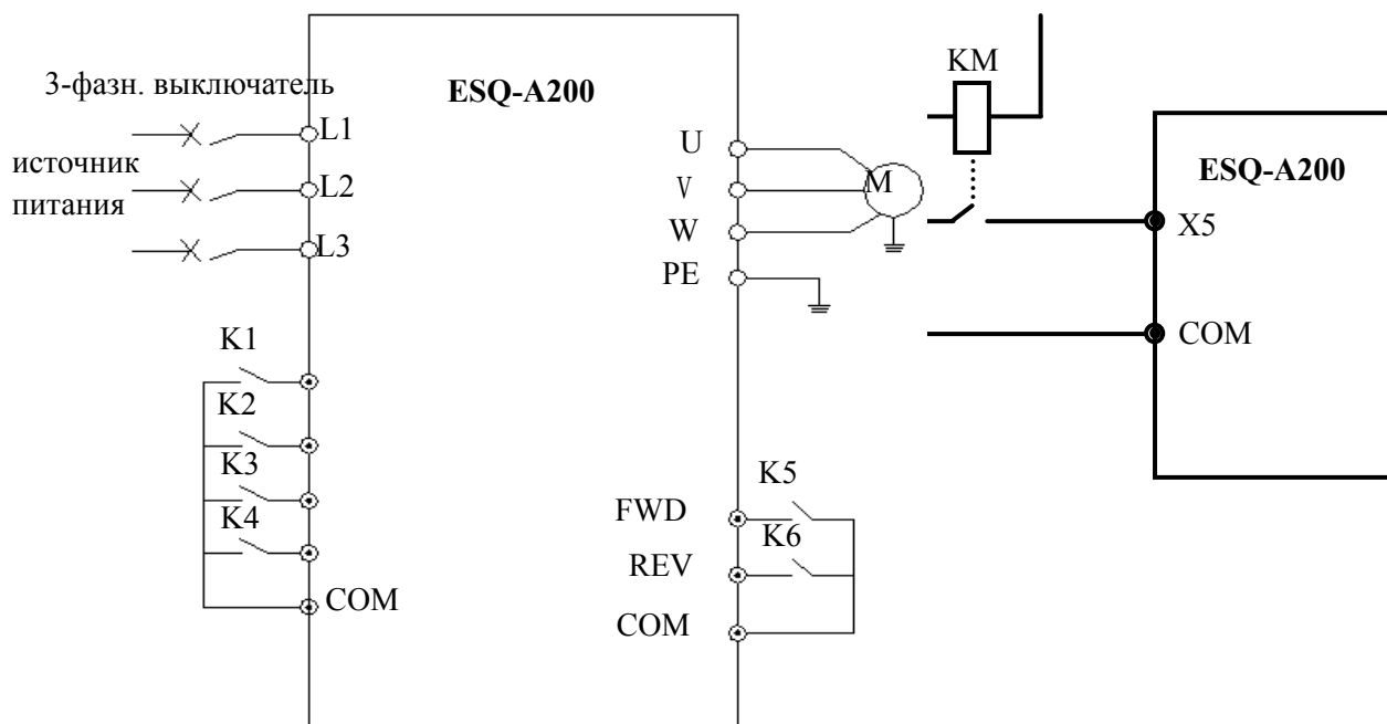
Рис.6-26 Работа на многоступенчатвой скорости
