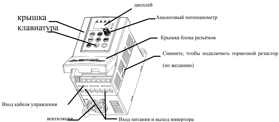
Рис. 2-2 Название деталей
