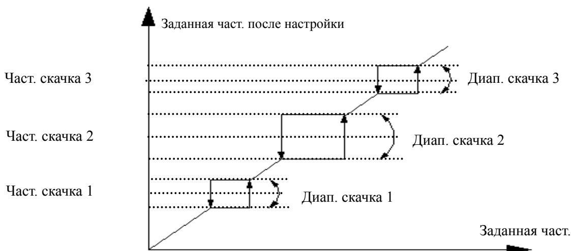
Рис.6-12 График частоты и диапазона скачка
