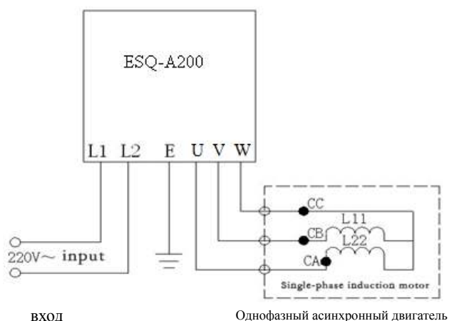
Рис.3-4 Способы подключения инвертора к двигателю
