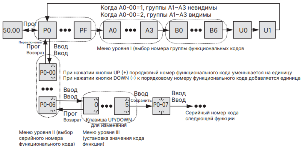
Меню уровня I (выбор номера группы функциональных кодов)
